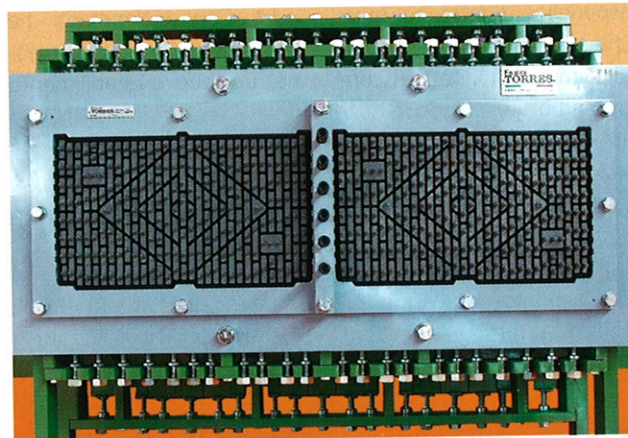
»4 Dettaglio della filiera per l'estrusione a larghe uscite di materiale a setti sottili
